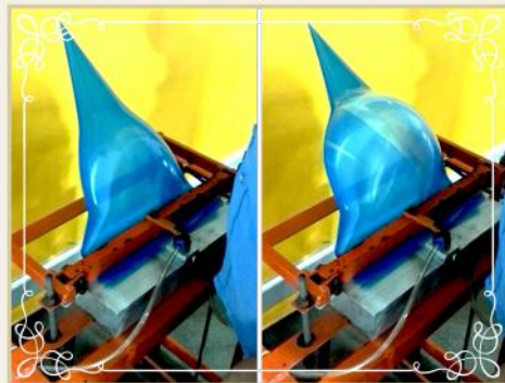
4. Ensayo de Resistencia Resistance Test
