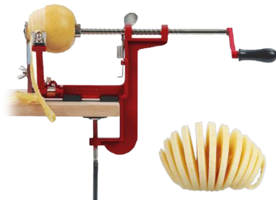
Pela manzanas con tornillo para mesa. Peel apples with table screw.
