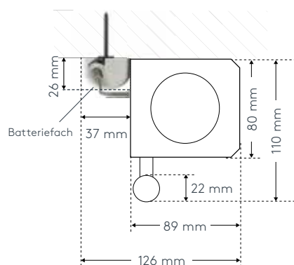
Deckenmontage D
