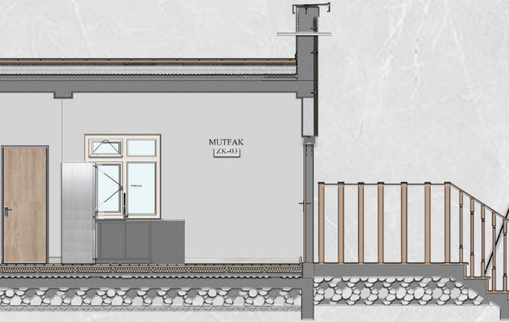
BB' KESİT 1\20
