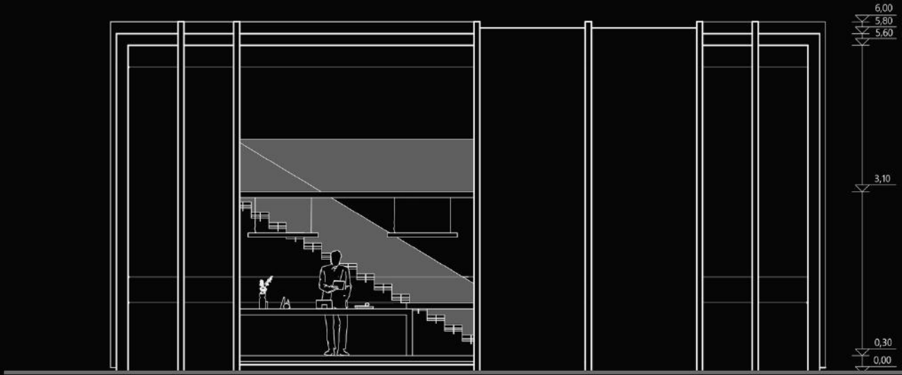
1\50 Ön Görünüş
