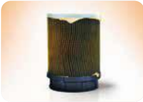
Diesel-Kraftstofffilter ohne Premium-Diesel ecoDrive nach 50.000 km
