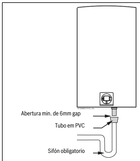
Fig. 25 Esquema de instalación de condensados
