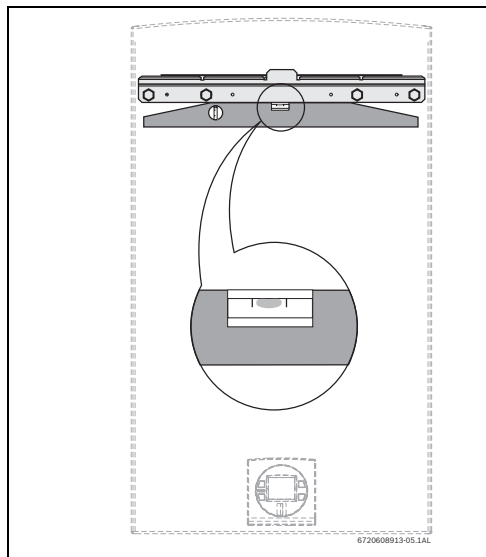
Fig. 20 Fijar la barra de fijación
