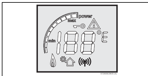
Fig. 12 Indicación de control remoto/mando a distancia
