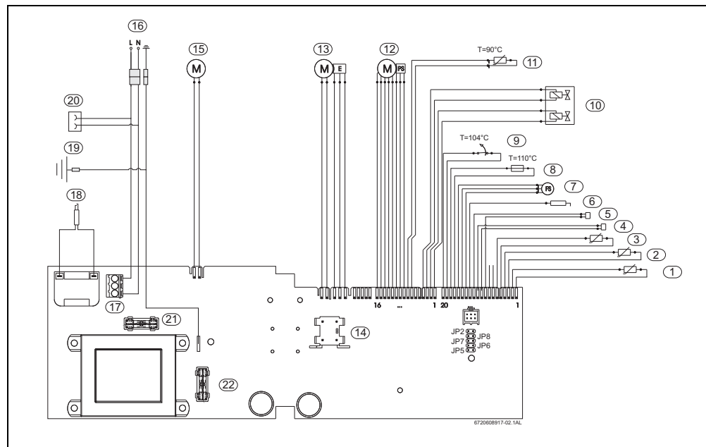
Fig. 3 Esquema eléctrico
