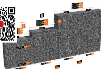
Réalisation d'un mur avec 3 hauteurs
