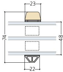
Lavenergisprosse 42 mm uden profil | NATic12-81L48
