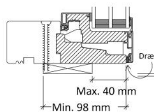
Bund montage gennem karm ved elementer under 150 kg
