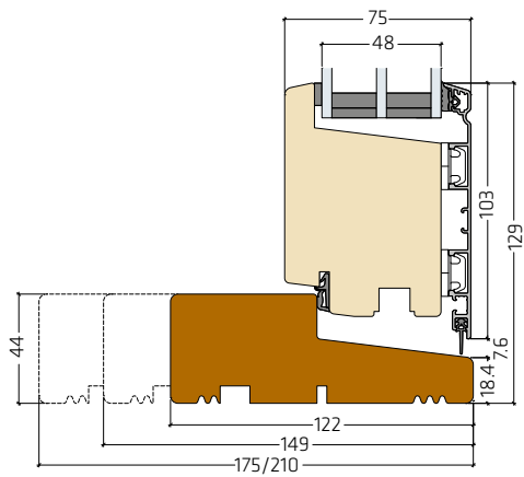
Hårdtræsbundtrin til udadgående facadedøre | FRAic21-10L48
