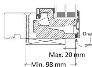
Bund montage gennem karm ved elementer over 150 kg
