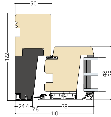
Hårdtræsbundtrin til indadgående facadedøre | FRAic22-10L48
