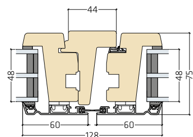
Sammenlukkende vinduesrammer | FRAic01-80L48
