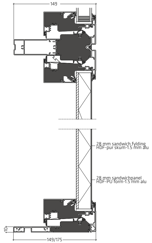
28 mm sandwich fyldning | PLU-FYL003
