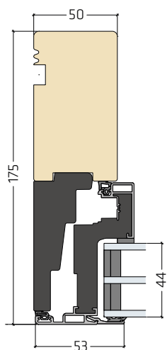
Alternativ karmdybde 50 x 175 mm | PLU01_30L44
