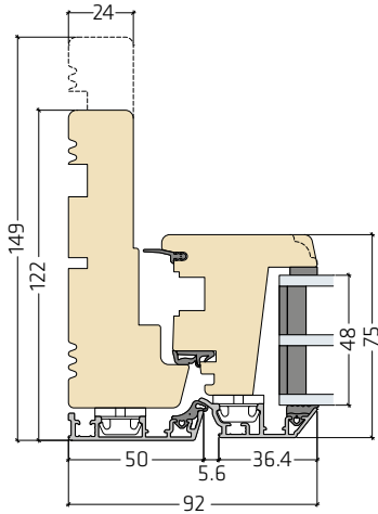
Karmdybde 122 og 149 mm | NATic09-30L48
