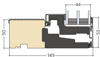
50 x 149 mm træbundkarm med alu-slidtrin | PLU20-10L44
