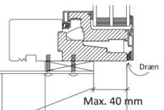
Bund montage med beslag ved elementer under 150 kg
