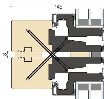
Sløjfeliste | PLU-PF0021
