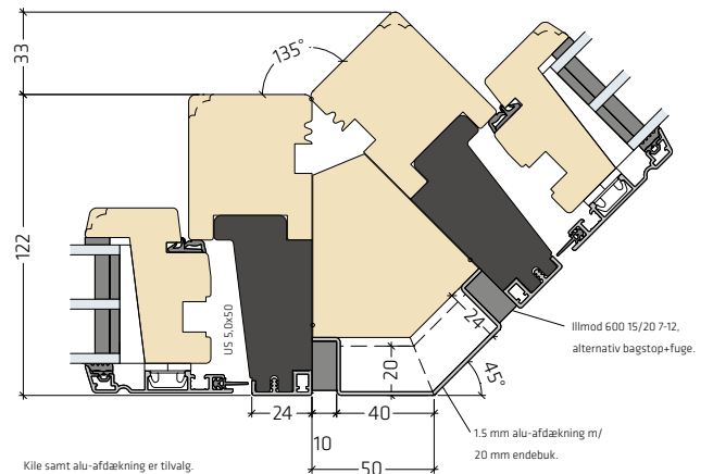
Hjørneløsning 45° med kile | FRAic-HJL013
