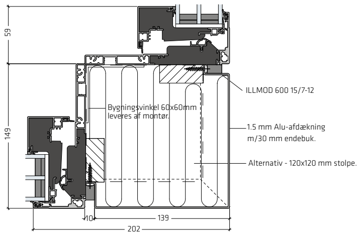
Hjørneløsning 90° uden fals | PLU-HJL030 Indadgående/indadgående
