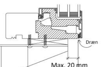
Bund montage med beslag ved elementer over 150 kg
