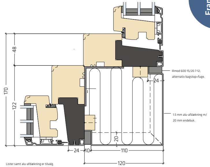
Hjørneløsning 45° med kile | FRAic-HJL013
