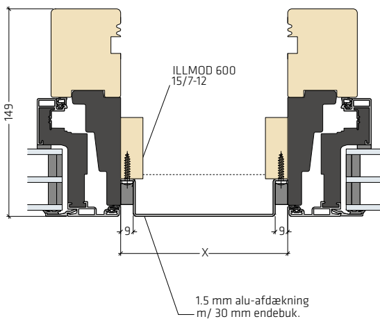
Hjørneløsning 180° inddækning | PLU-HJL011
