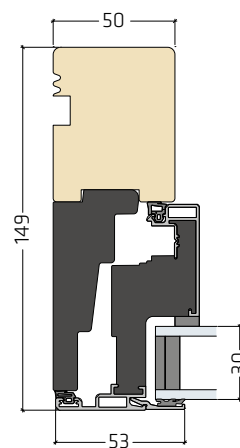
Sidekarm med 2-lags rude | PLU01-30L30
