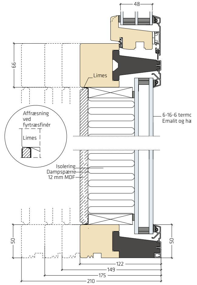
Fuldt isoleret brystning med emalitglas | FRAic-FYL004
