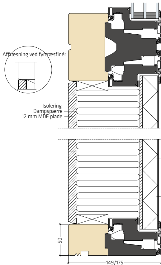
Fuldt isoleret brystning med sandwich fyldning | PLU-FYL020
