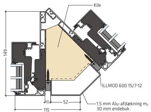
Hjørneløsning 45° med kile | PLU-HJL032 Indadgående/indadgående
