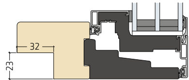
23 x 32 mm fals ved udskiftning | PLU-NOT006
