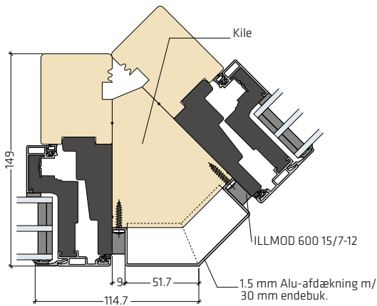
Hjørneløsning 45° med kile | PLU-HJL005
