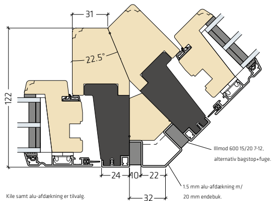
Hjørneløsning 45° med smigskæring | FRAic-HJL009
