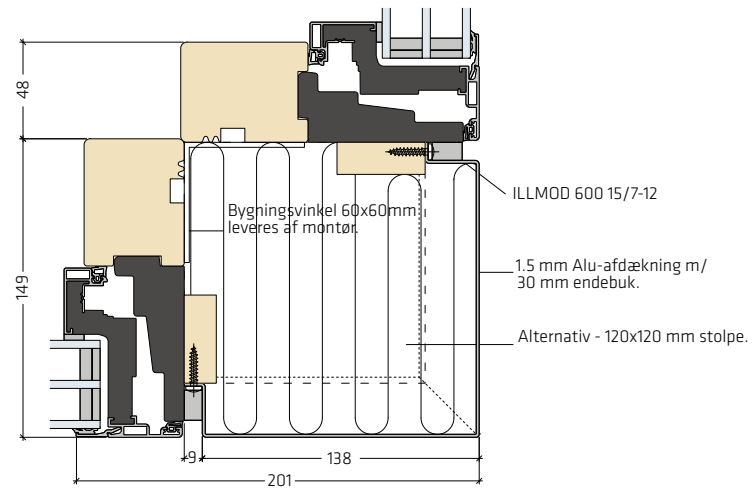
Hjørneløsning 90° uden fals | PLU-HJL003
