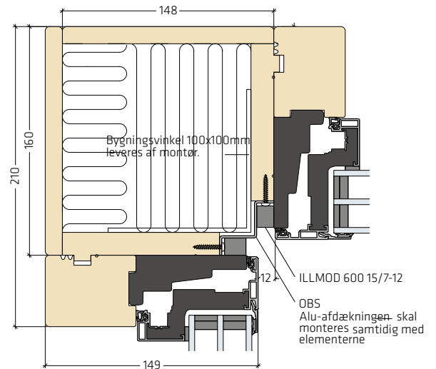
Hjørneløsning 90° med indadgående hjørne | PLU-HJL009
