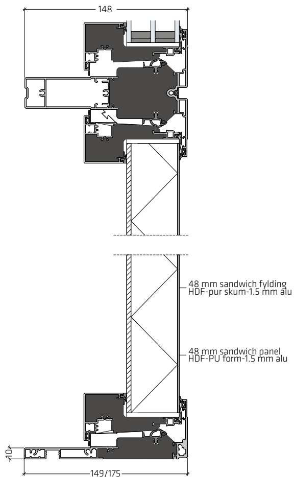
48 mm sandwich fyldning | PLU-FYL002
