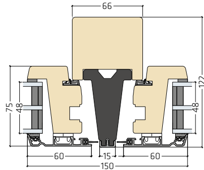
66 x 122 mm lodret post med rammer | FRAic01-50L48
