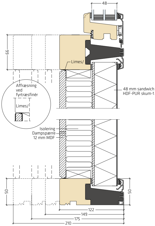
Ventileret og fuldt isoleret brystning | FRAic-FYL005
