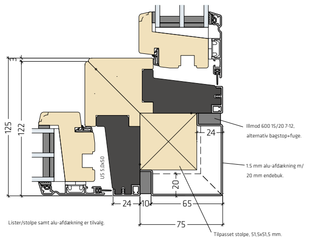
Hjørneløsning 90° med smigskæring | FRAic-HJL018
