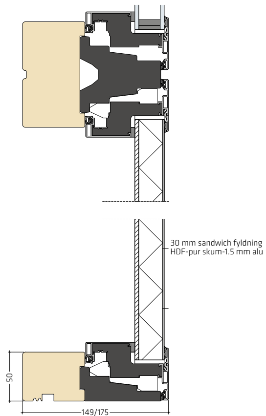
Fuldt isoleret brystning med termorude | PLU-FYL030
