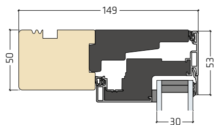
Topkarm med 2-lags rude | PLU01-20L30
