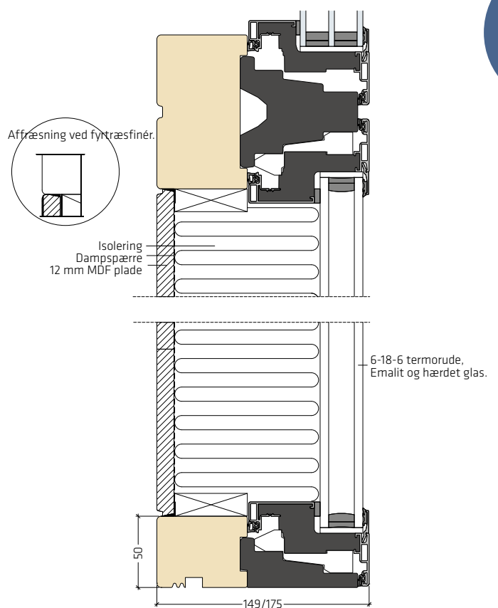
Fuldt isoleret brystning med termorude | PLU-FYL030
