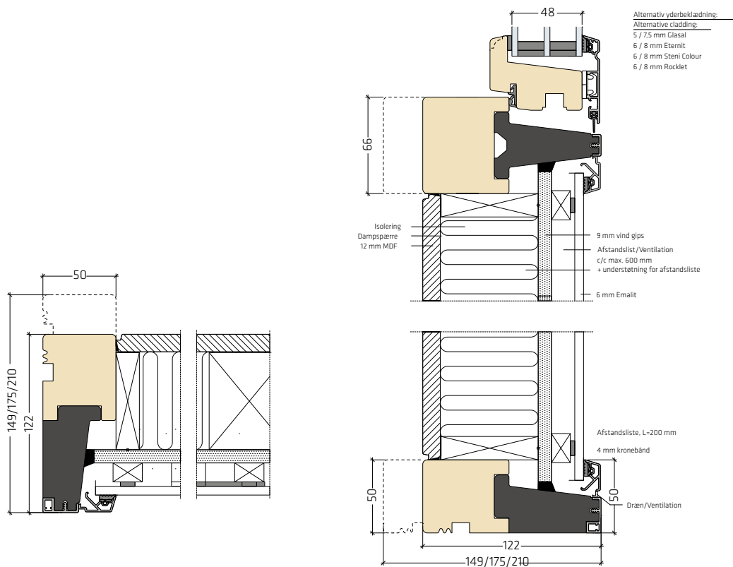
Ventileret og fuldt isoleret brystning | FRAic-FYL005
