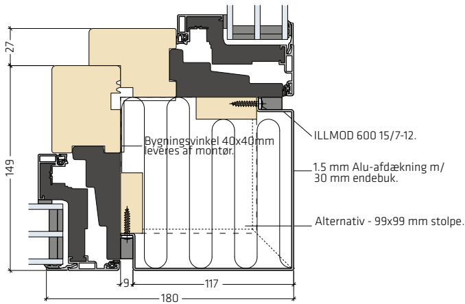
Hjørneløsning 90° med fals | PLU-HJL001
