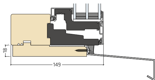
Påforing til montage af vandnæser | PLU-PF0001
