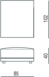
POUF OTTOMAN 85 X 102
