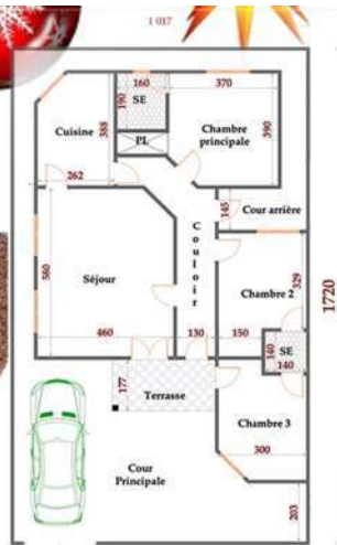
VUE EN PLAN COTEE
