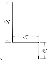
44 ABS Sidewall (ABSSWcc)
