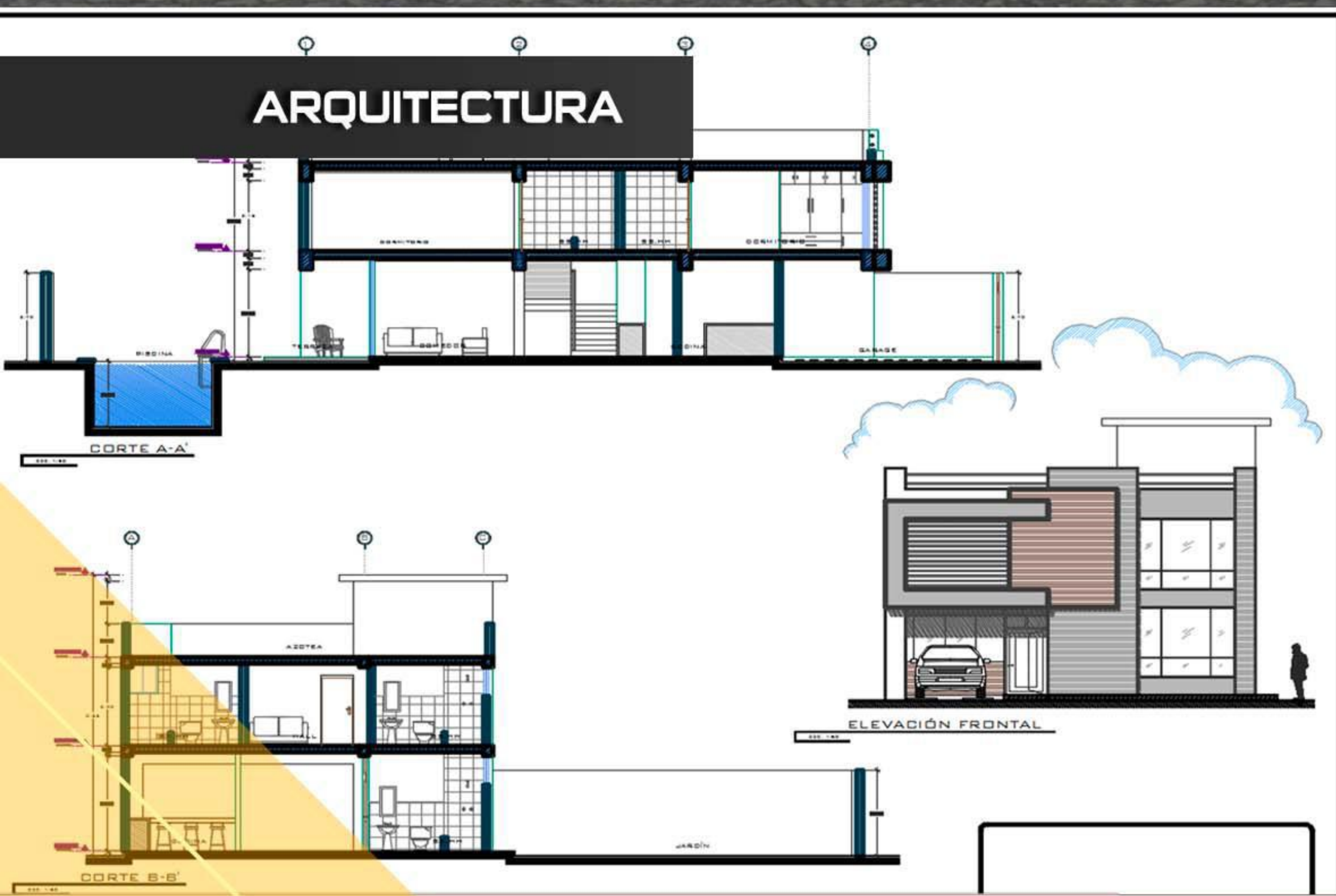
DISEÑO INTEGRAL DE VIVIENDA UNIFAMILIAR
