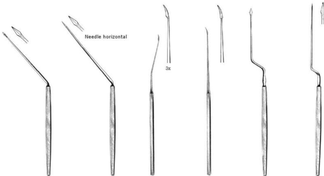
Politzer 21-184-16 16.5 cm/ 6½"
