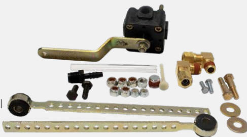
Válvula control de altura bombonas.
